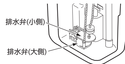
排水弁(小側)
