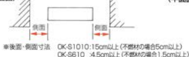
〈平面図〉
