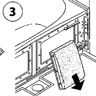
下部から取り外す
