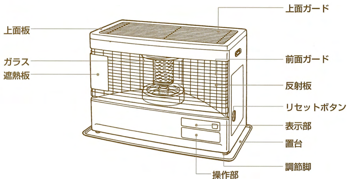
【正面外観図】
