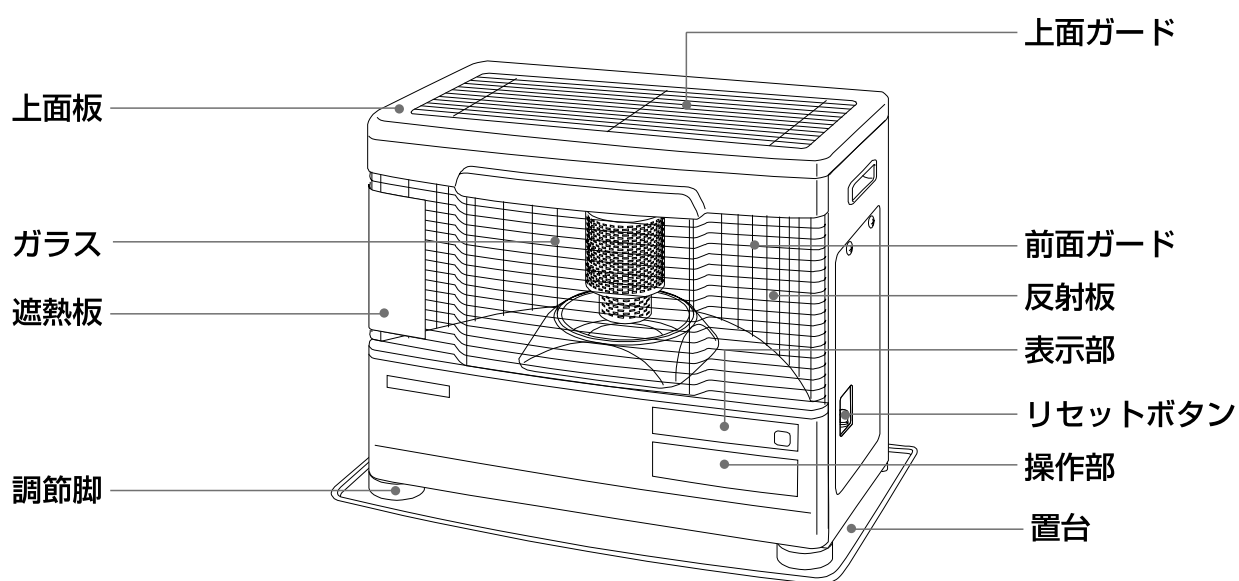
【正面外観図】
