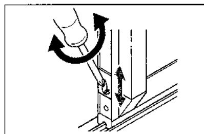
戸車調節ねじ
