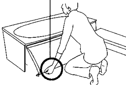
手かかりの奥にあるクリップを指で 押さえながら浴槽のセキに乗せる
